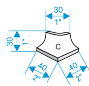
Narożnik zewnętrzny Foot
