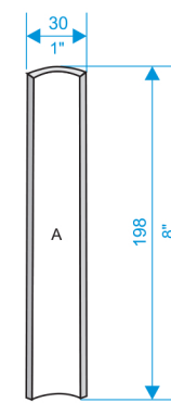
Profil wklęsły Inside bead
